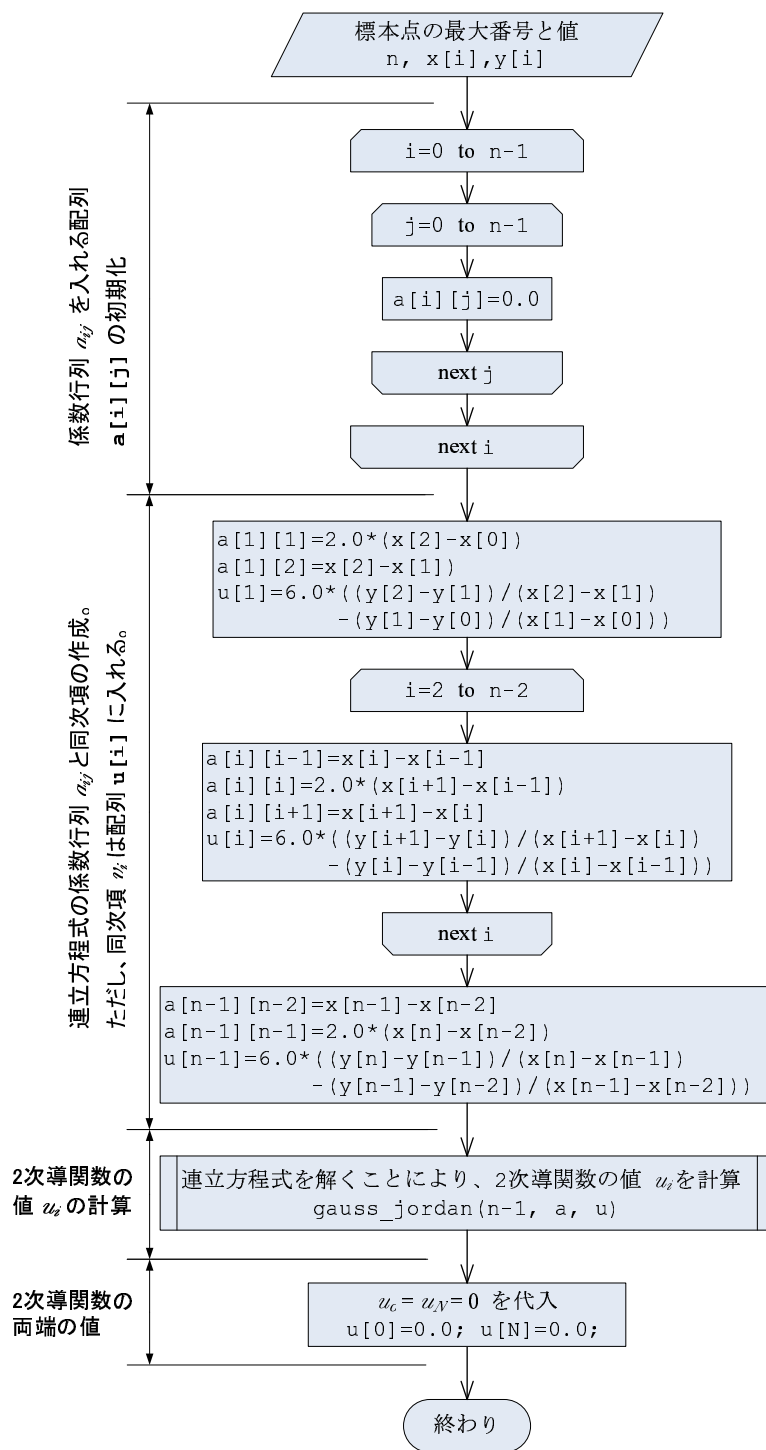
図 1: 2次導関数 u_i を求める関数 .
