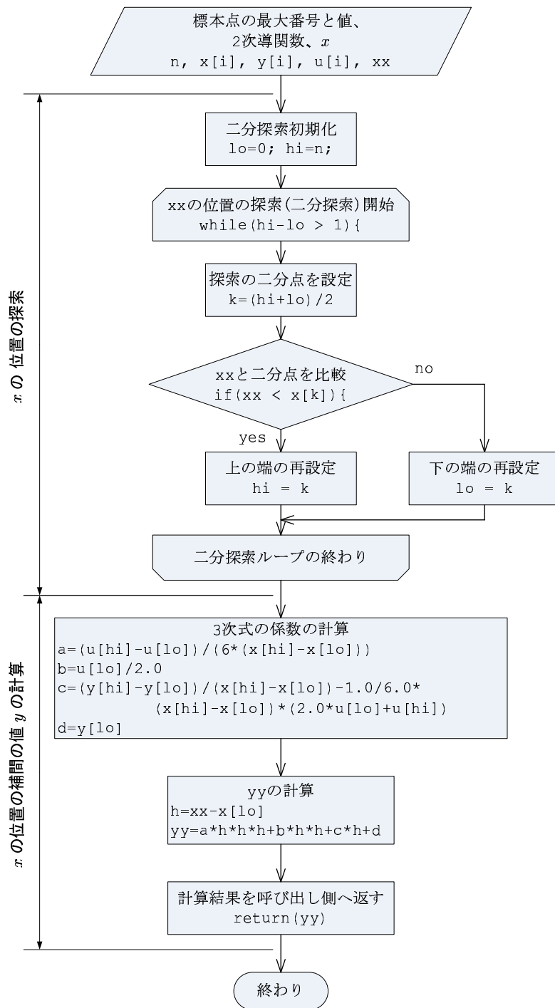
図 2: 補間された値を求める関数 .
